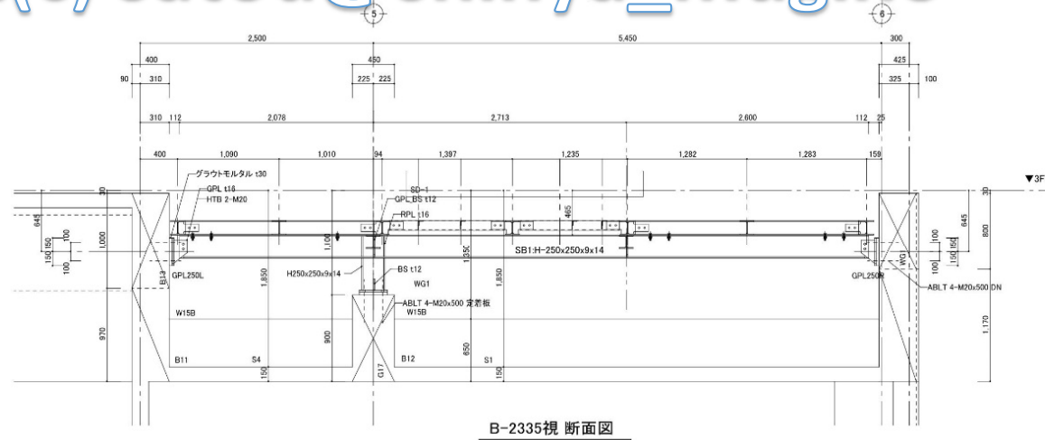
B-2335 視断面図
